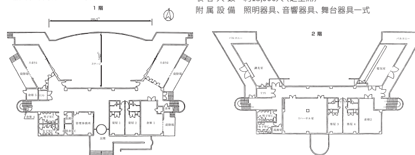
稲佐山公園野外ステージ平面図 縮尺 1:200
